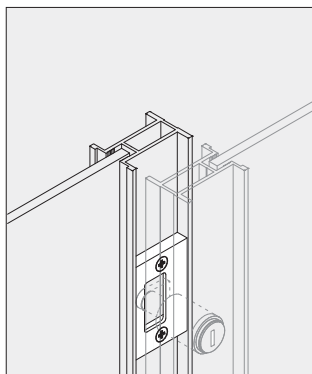
Schließblech auf dem hinten liegenden Rahmen
