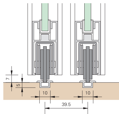
Art.-Nr. 318 Laufschiene zum Einlassen
