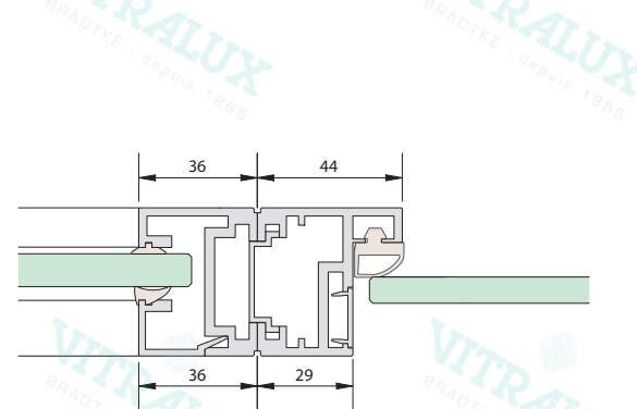
MR 36 Rahmen und AT 44 Anschlagtürzarge mit Easy-Connection
