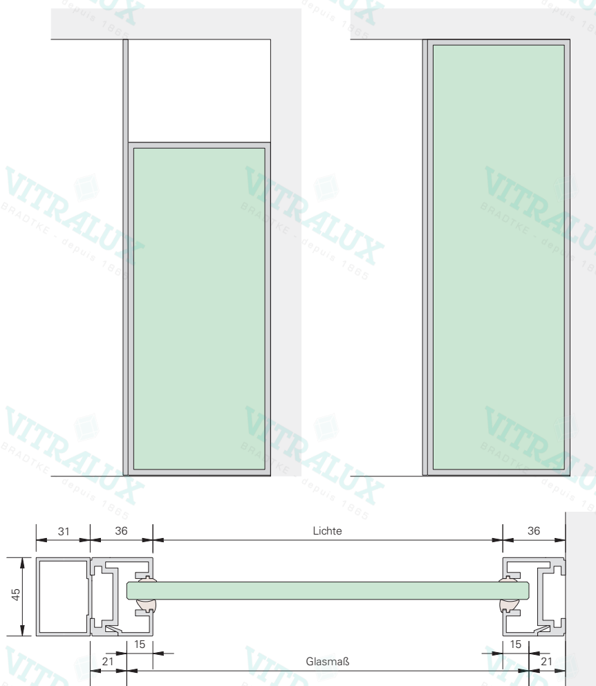
MR 36 kombiniert mit Zusatzprofil 31/45 freistehende Rahmen als Abschluss und Deckenanschluss
