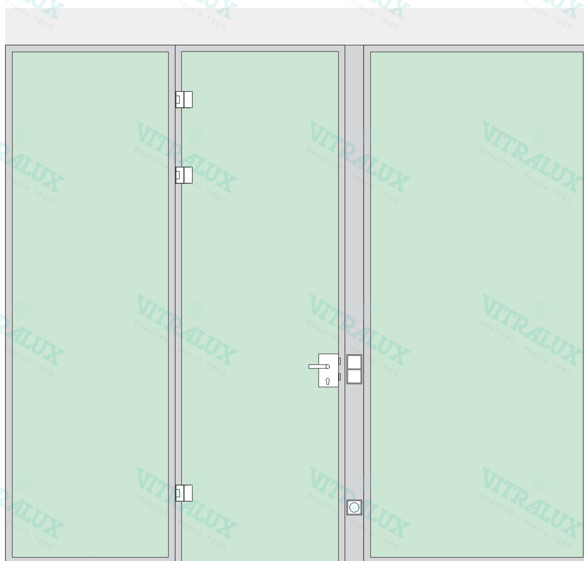
Rahmen Typ 100
