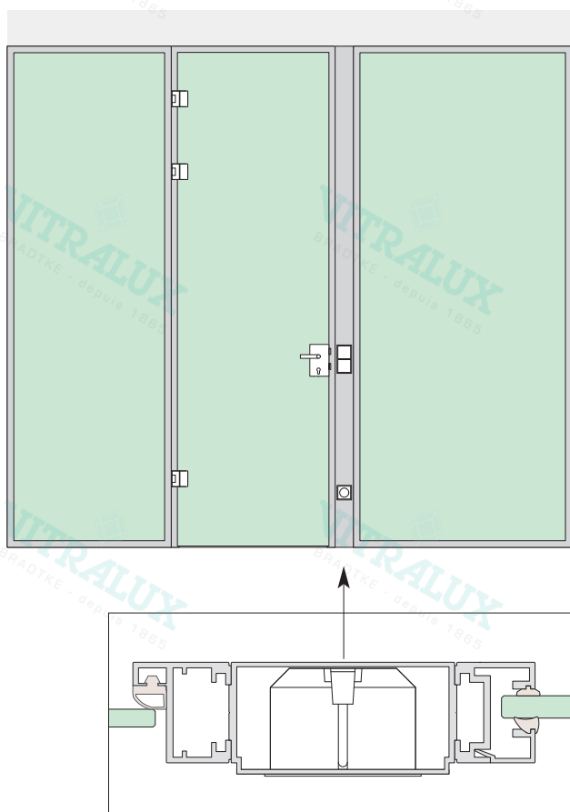
Zusatzpaneel für Elektroinstallation
