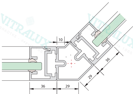
MR 36 Rahmen mit 135 Grad Eckprofil
