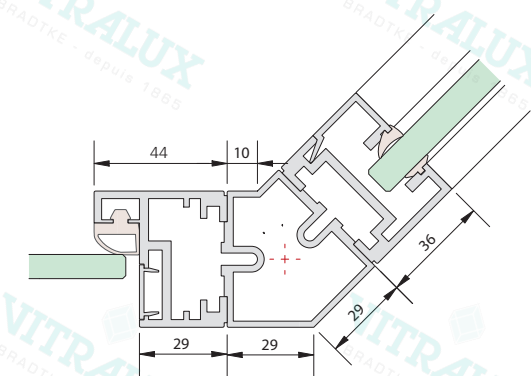
AT 44 mit 135 Grad Eckprofil
